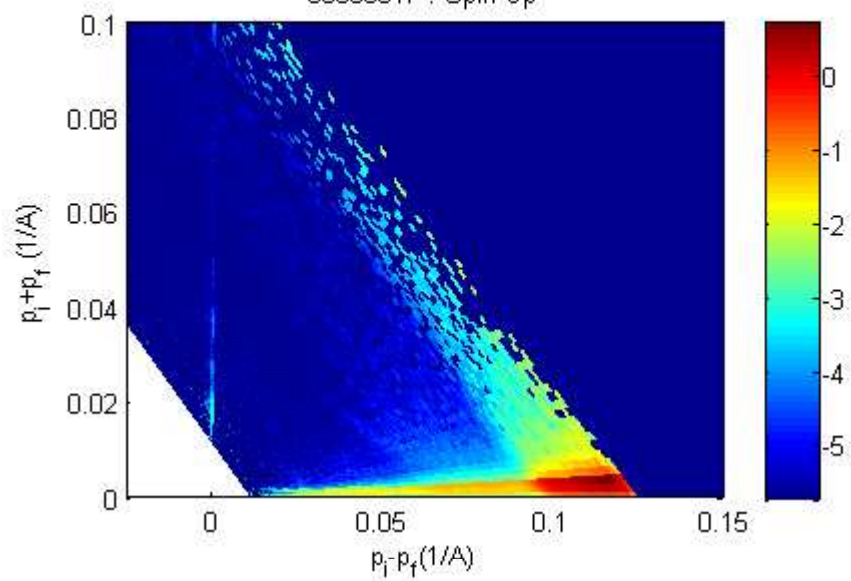
00006017 : Spin Up
